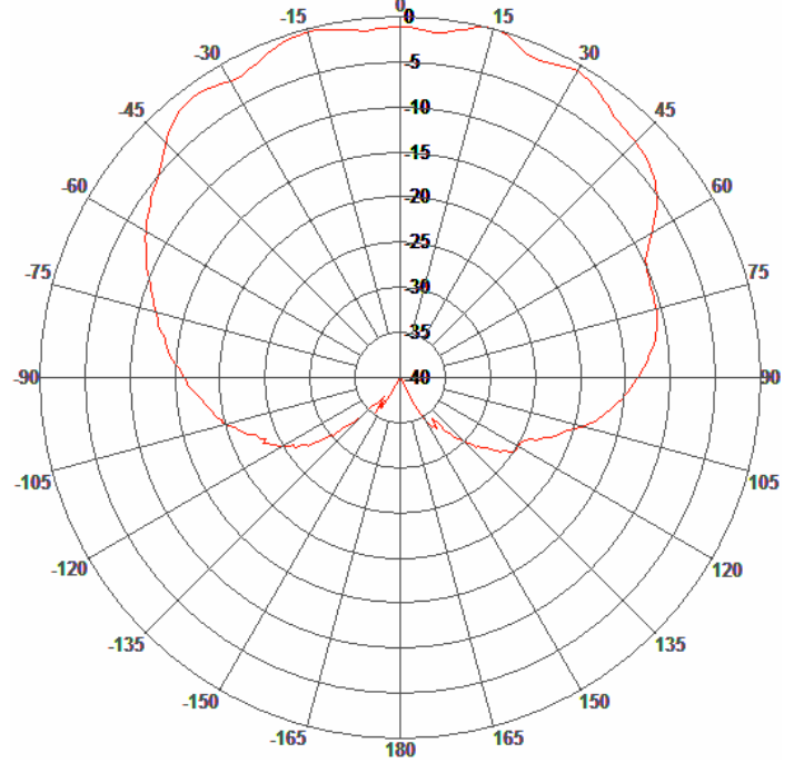
H-Plane Pattern
