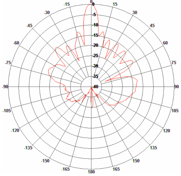
H-Plane Pattern
