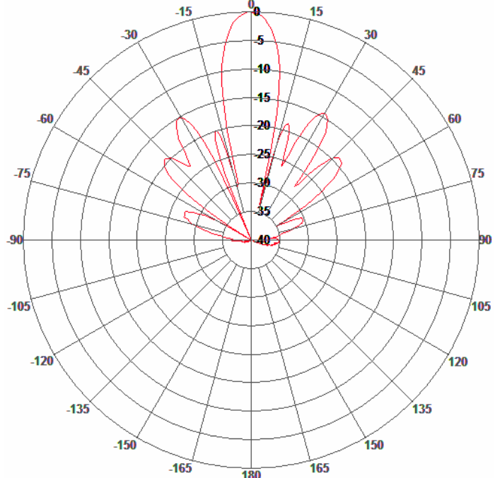
H-Plane Pattern
